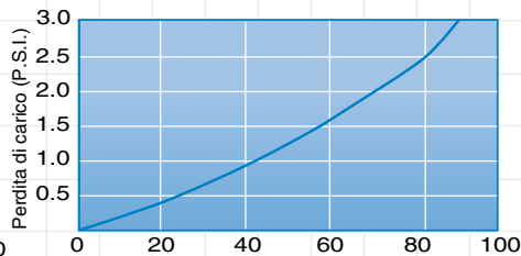
Perdita di carico WB 90SC-2
