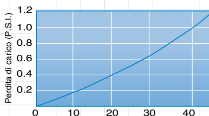
Perdita di carico WB 40SC-2
